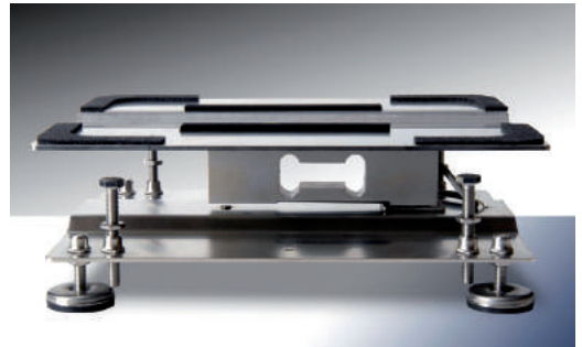
Detail der Konstruktion
